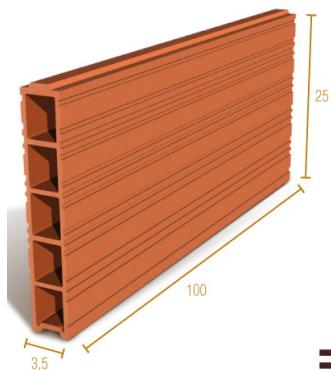
BARDO 100X25X3,5
