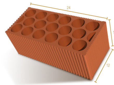
MACIZO PANAL 24X12X10 3ª
