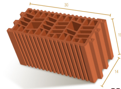
TERMOCERAMICA 30X19X14
