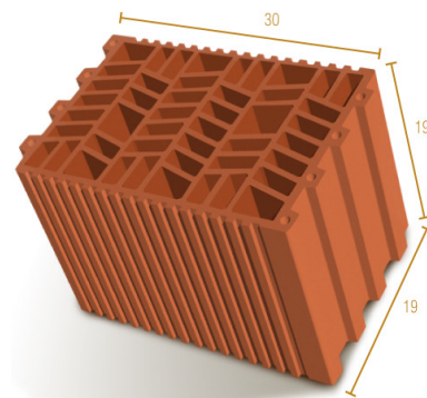
TERMOCERAMICA 30X19X19
