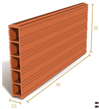
BARDO 80X25X3,5
